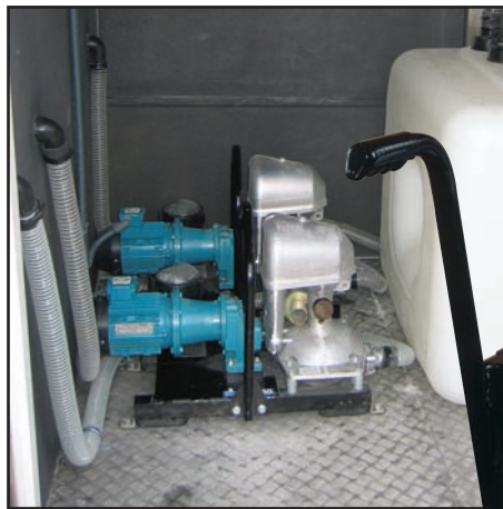
Pumpanlage auf Freizeitboot (Großbritannien)
